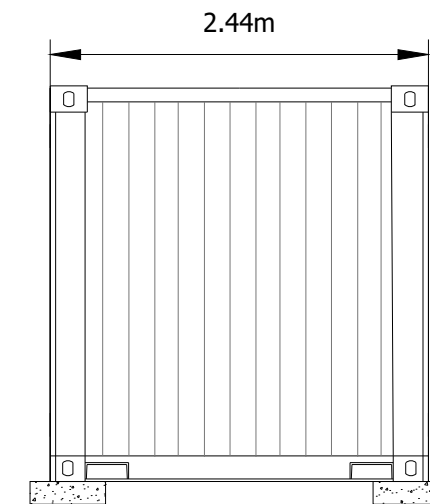
END ELEVATION
